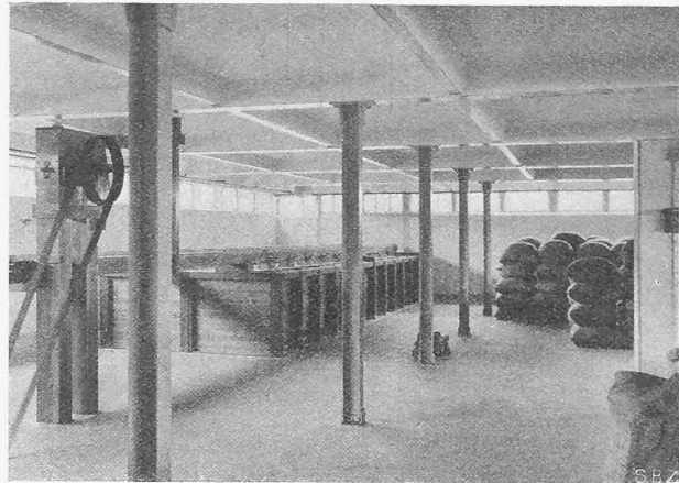
Abb. 2. Oberstes Halbgeschoss mit Dach-Untersicht.
